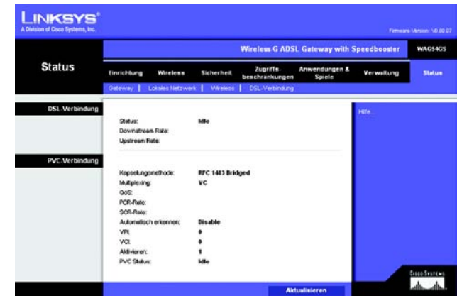
Abbildung 6-47: DSL-Verbindung
